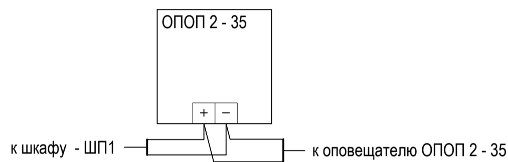
Типовая схема подключения оповещателя ОПОП 2 - 35
