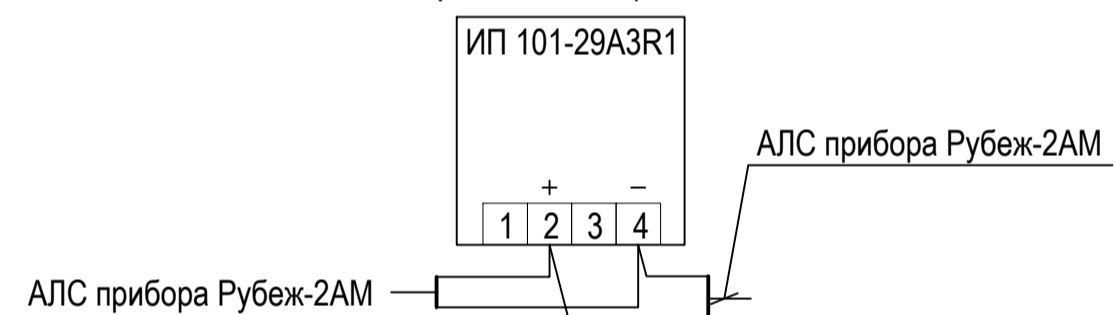
Типовая схема подключения теплового пожарного извещателя ИП 101-29А3R1 к АЛС
