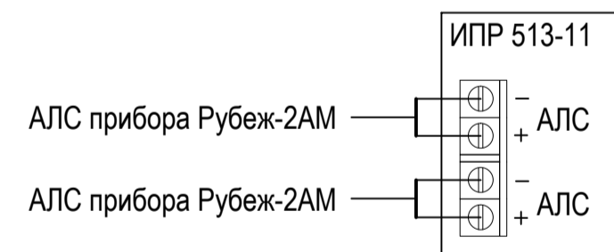
Типовая схема подключения извещателя ИПР 513-11 к АЛС
