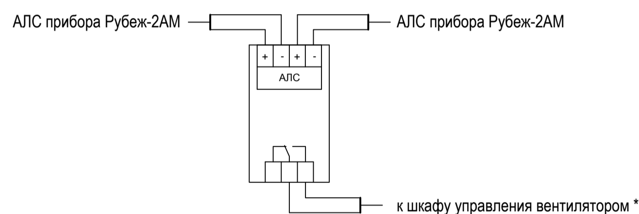
Типовая схема подключения релейного модуля РМ - 1
