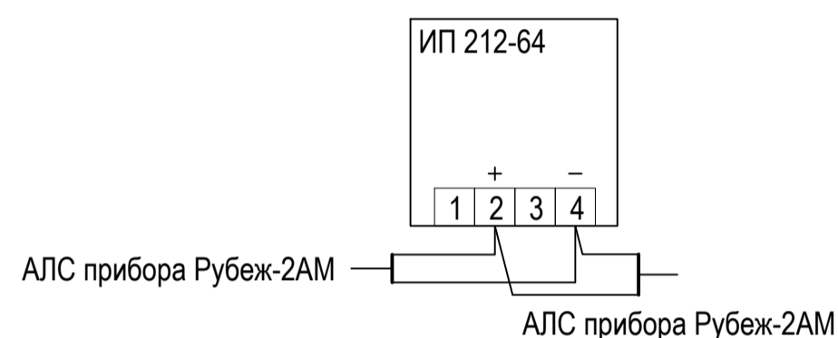
Типовая схема подключения извещателя ИП212-64 к АЛС
