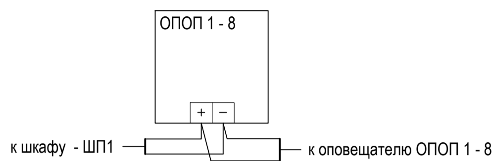
Типовая схема подключения оповещателя ОПОП 1 - 8
