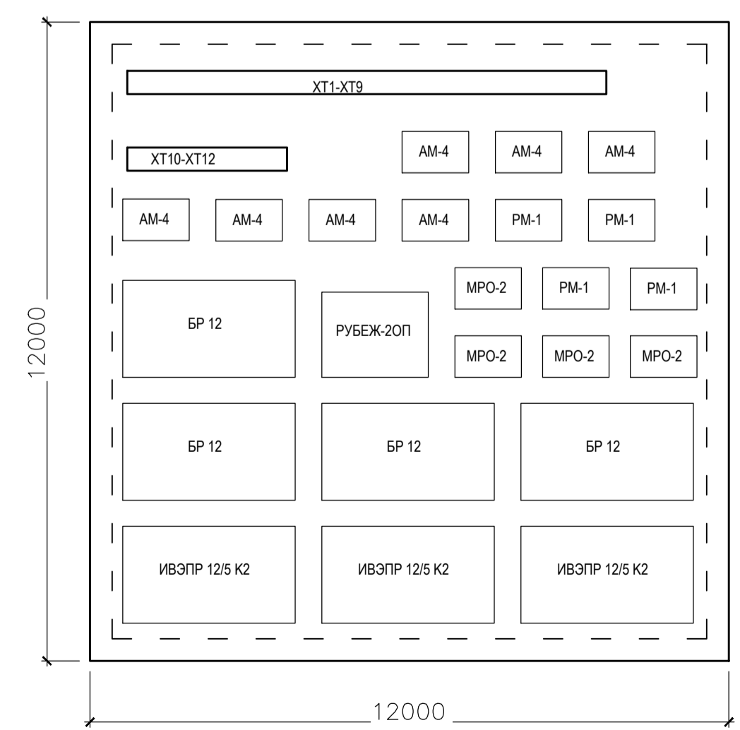
ШП 1 Чертеж общего вида
